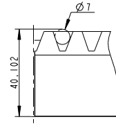
SCALE 5:1
