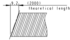
SCALE 5:1
