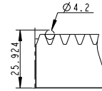
SCALE 5:1
